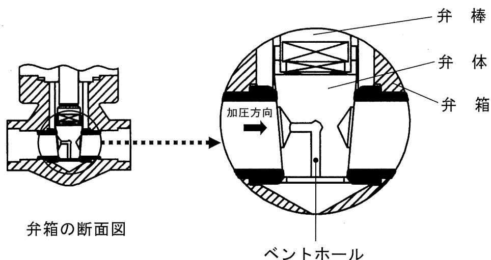
図 1.1 ベントホール（ディスクホール）
