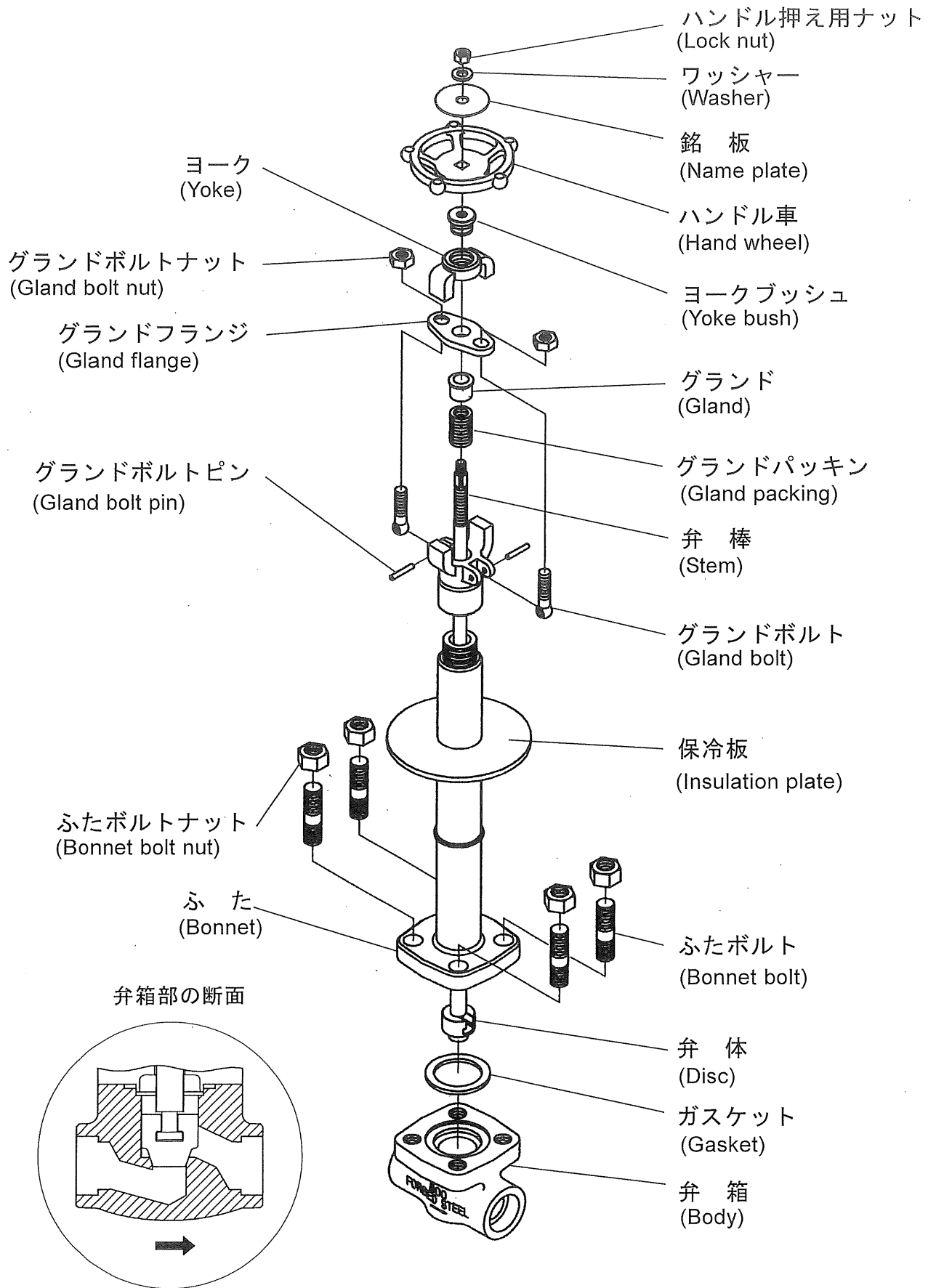
図 2.2 クラス 800 玉形弁の代表的な例
