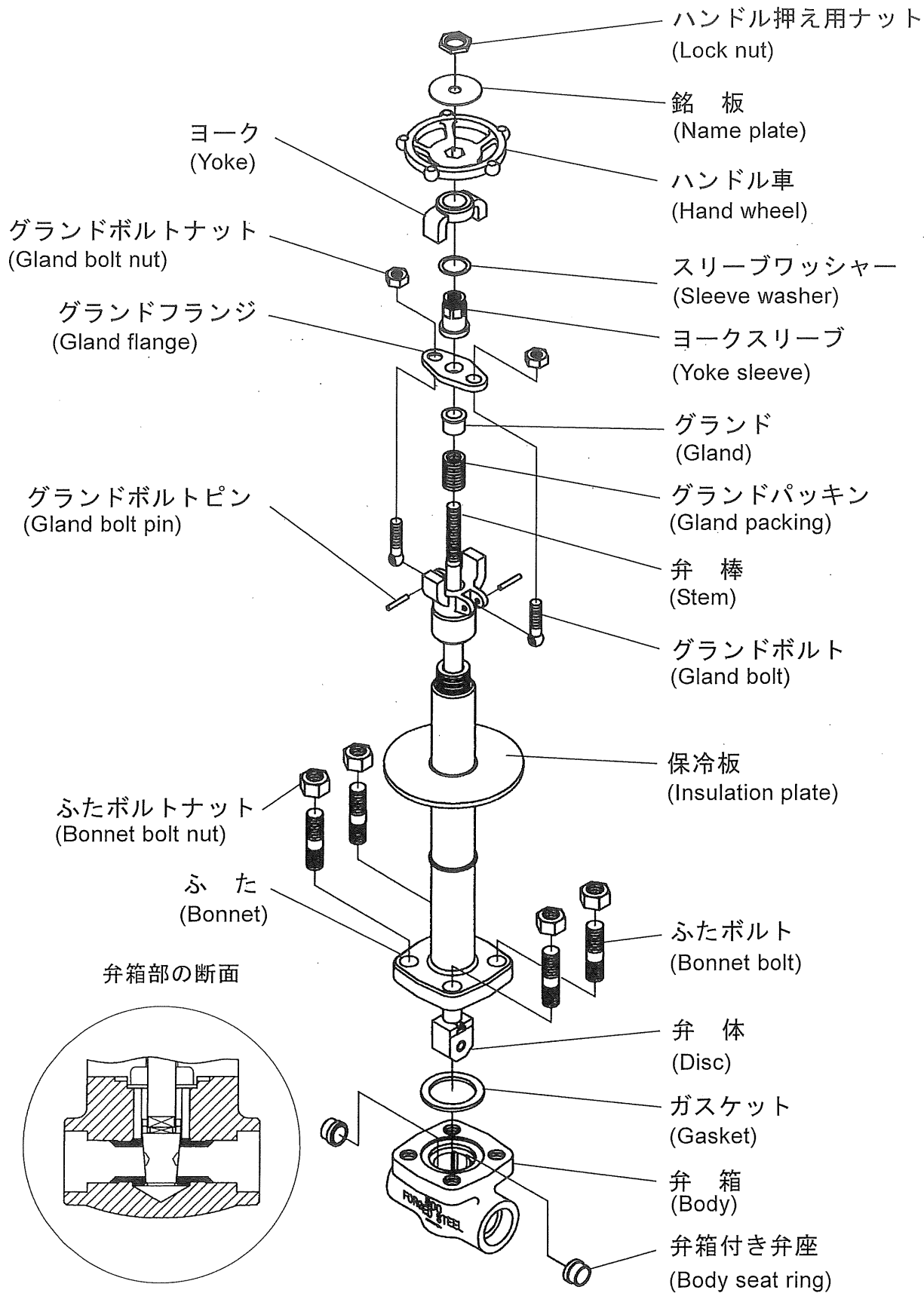
図 2.1 クラス 800 仕切弁の代表的な例
